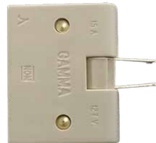
CLAVIJA TRIPLE BISAGRA CUERPO DE BAQUELITA HERRAJE DE LATÓN 15A/127V
